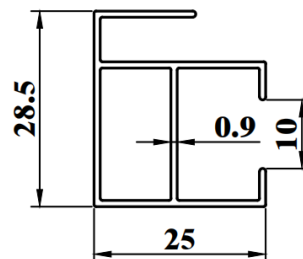
SW700A WEIGHT : 0.290 KG/M AP : 176.75mm
