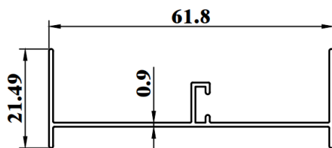
SW697A WEIGHT : 0.287 KG/M AP : 234.61mm
