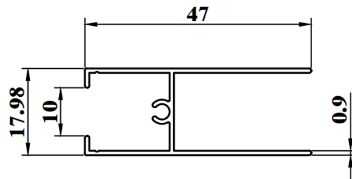
SW699A WEIGHT : 0.303 KG/M AP : 244.49mm
