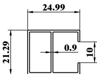
SW701A WEIGHT : 0.240 KG/M AP : 135.52mm
