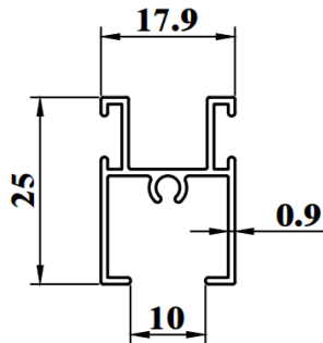
SW698A WEIGHT : 0.228 KG/M AP : 179.46mm
