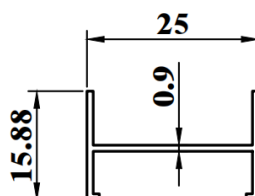
SW702A WEIGHT : 0.138 KG/M AP : 115.32mm
