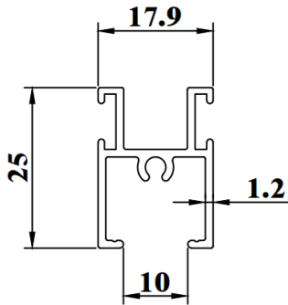
SW698G WEIGHT : 0.288 KG/M AP : 177.13mm
